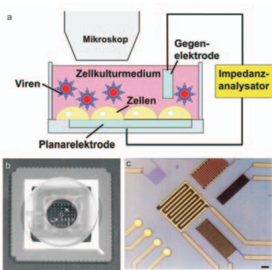
Abbildung 1: Chipbasierte Bestimmung des virusbedingten cytopathischen Effekts auf Zellen. a: Schematische Darstellung des Messprinzips. b: Multielektroden-Chipeinheit mit Kulturschale. c: Lichtmikroskopische Aufnahme von verschiedenen Elektrodenstrukturen für die Impedanzmessungen.
