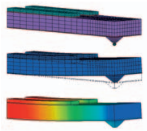
Abbildung 3: Modell, Verbiegung und Auslenkung des mit einer Referenzkugel (42 µm Durchmesser) belasteten Werkzeugs.
